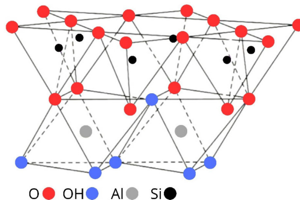
Figura 3: Exemplo de estrutura cristalina da caulinita. Fonte: Elaboração própria.
